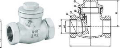
旋启式内螺纹止回阀
