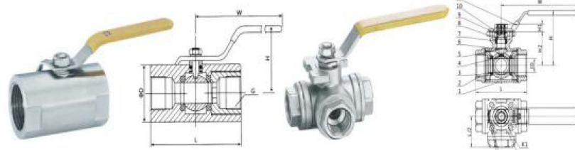
广式内螺纹球阀
