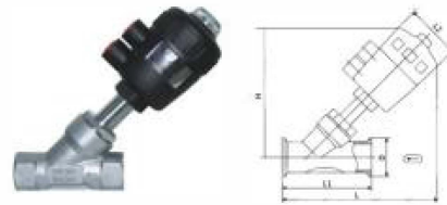
气动角座阀
