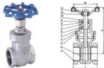
不锈钢内螺纹闸阀
