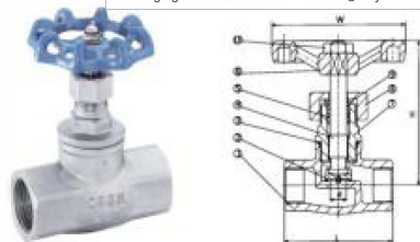
不锈钢内螺纹截止阀
